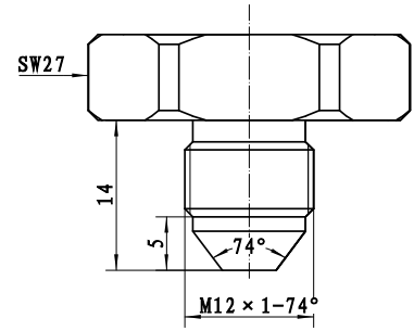
M12×1 Male, 74° cone (C14)
