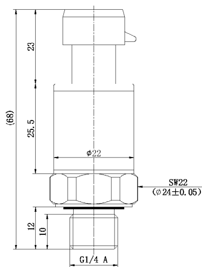
B5(Packard)
